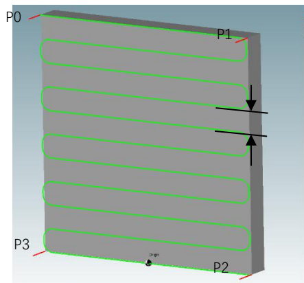
左图给出了机器人执行的轨迹示例。
